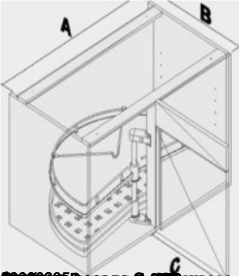
100002053 Артикул А 1000 мм, диаметр 450 мм, высота 200 мм, ширина 510 мм, дверца
